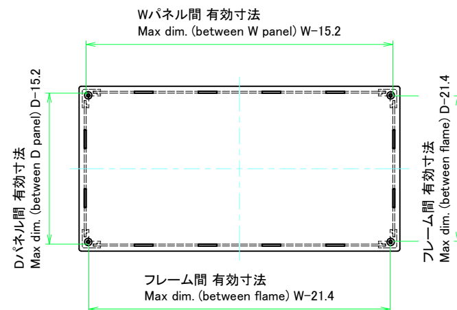
下カバー / Bottom cover
