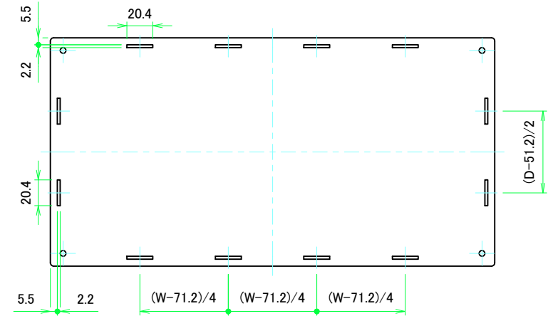
上カバー裏面 / Top cover Backside
